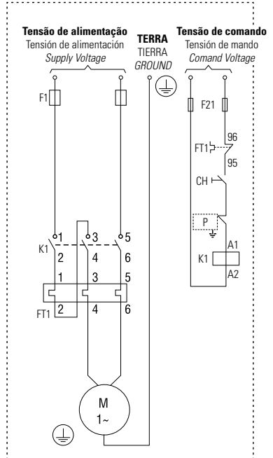
2 ESQUEMA DE CONEXÃO ELÉTRICA MONOFÁSICA (MOTOR STANDARD) ESQUEMA DE CONEXIÓN ELÉCTRICA MONOFÁSICA (MOTOR STANDARD) ELECTRICAL CONNECTION DIAGRAM (STANDARD MOTOR)
