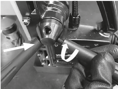
Fig. 5 – Montaje de la manivela
