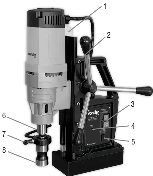
Fig. 1 – Componentes
