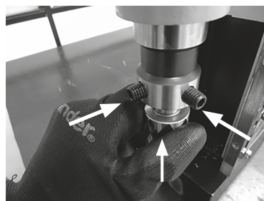
Fig. 4 – Instalação da broca
