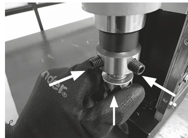
Fig. 4 – Instalación de la broca
