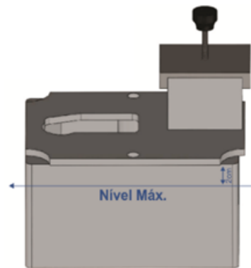
Figura 14 - Reservatório coleiro
