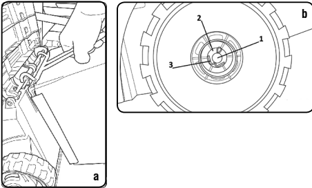
Fig. 3 – Montaje de la rueda
