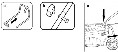
Fig. 2 – Instalação da alça
