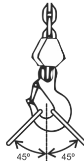
Fig. 3 – Uso de lingas
