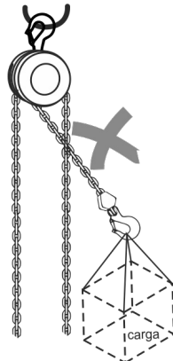
Fig. 2 – Movimiento de la carga
