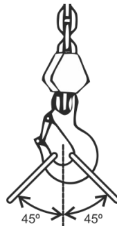
Fig. 3 – Uso de eslingas
