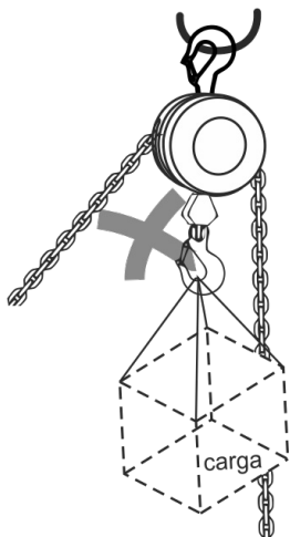
Fig. 4 – Elevação da carga
