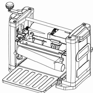
Fig. 3 – Montaje del extractor de polvo
