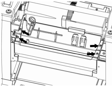
Fig. 14 – Removendo a proteção das lâminas
