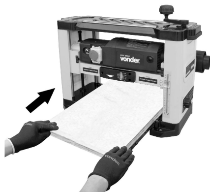
Fig. 8 – Posición segura de trabajo
